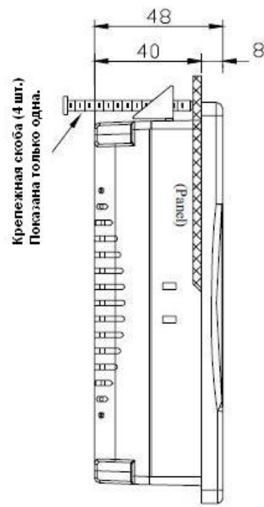
Вид сбоку
